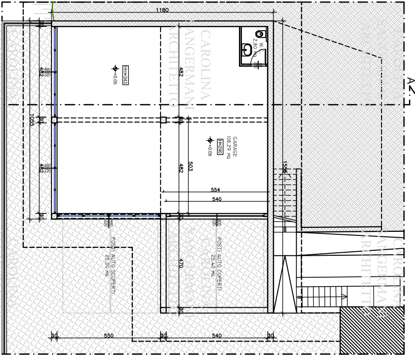
PIANTA PRIMO LIVELLO (GARAGE)
