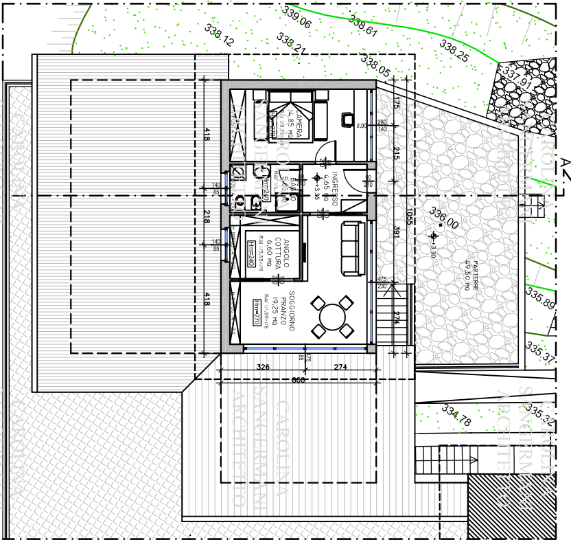
PIANTA SECONDO LIVELLO (ABITAZIONE)
